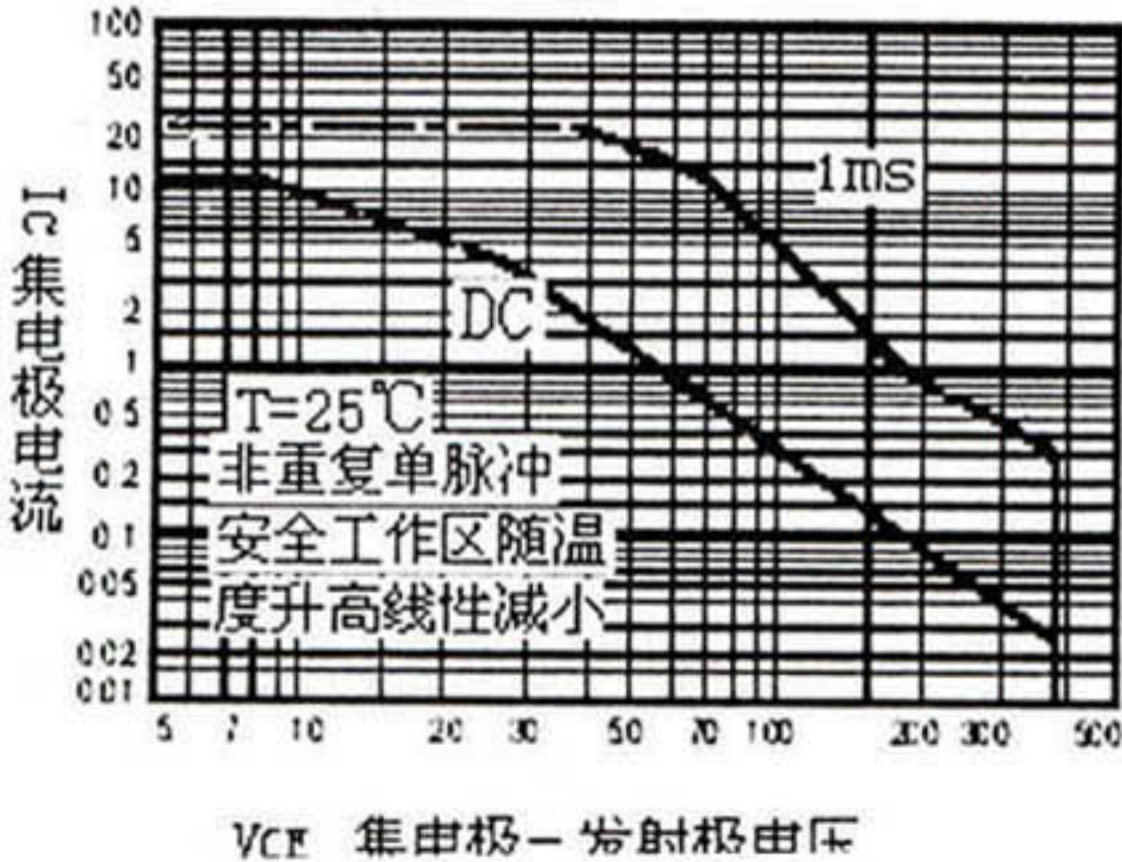
安全工作区
